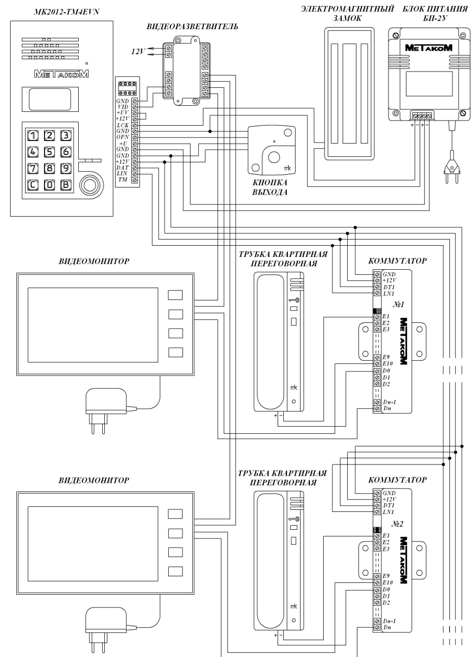
Рис. 2 Пример монтажа блока вызова МК2012-ТМ4ЕVН
